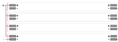
Параллельное подключение
